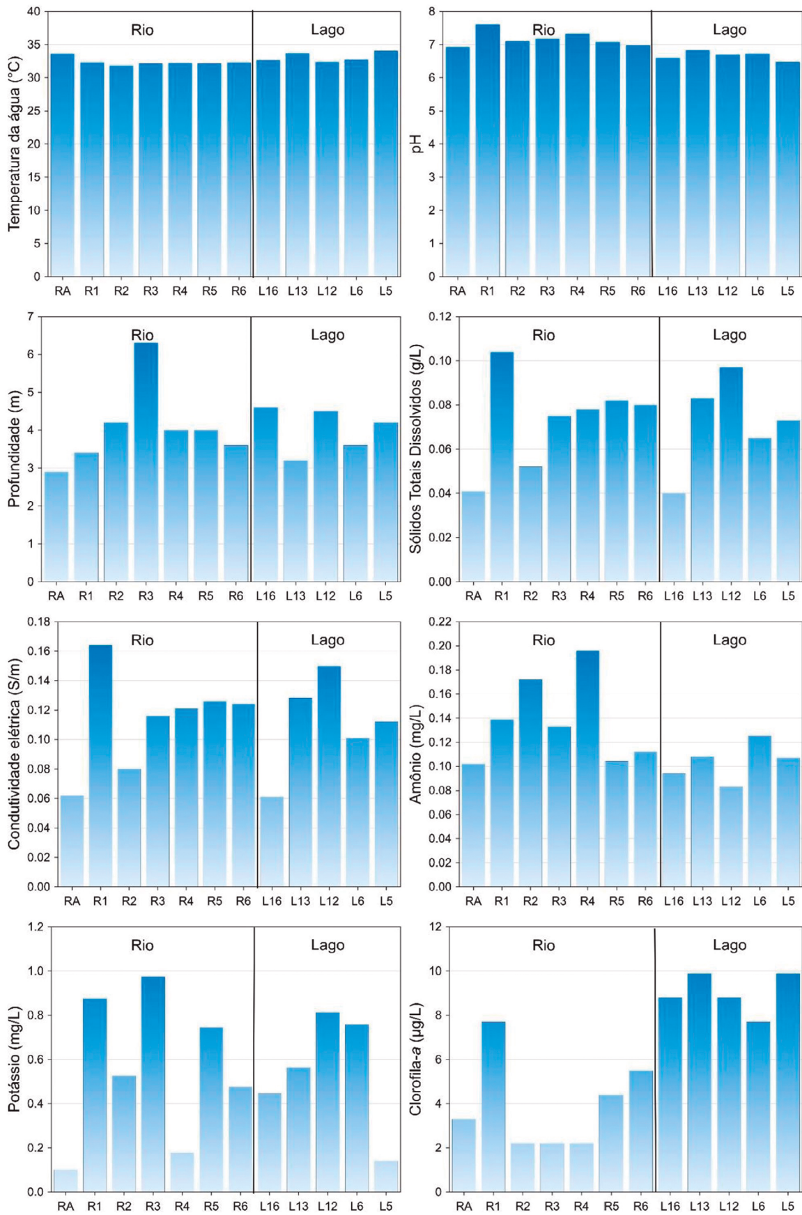
Figura 6. Variáveis ambientais levantadas em março de 2024, nos rios Vermelho e Araguaia, que apresentaram os menores Coeficientes de Variação nos ambientes fluviais (R1 a R6) e lacustres (L5 a L16). Por se tratar de outro sistema fluvial, o ponto de amostragem no Rio Araguaia (RA) não foi considerada para o cálculo dos Coeficientes de Variação.
